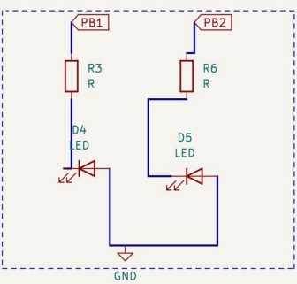
LED(s) contrôlé(e)s par microcontrôleur
