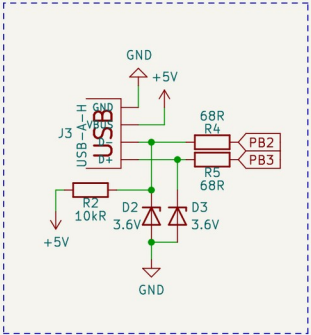
Connecteur USB
