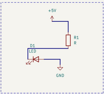
LED témoin de tension
