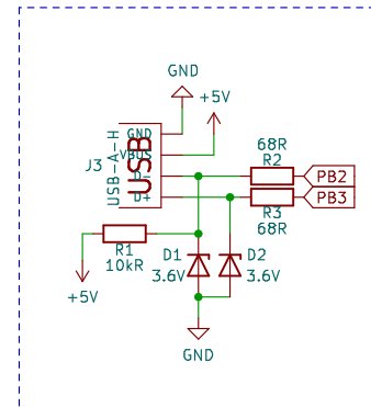
Connecteur USB
