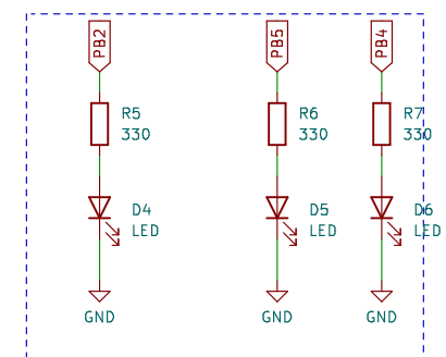
LED(s) contrôlée(s) par microcontrôleur
