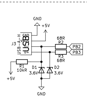
Connecteur USB
