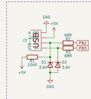
Connecteur USB
