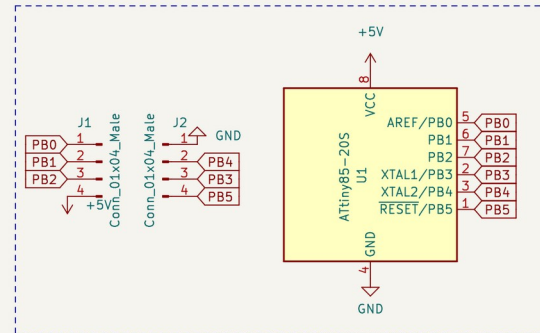
Partie microcontrôleur et broches de programmation
