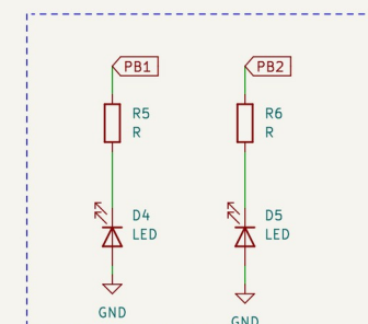
LED(s) contrôlée(s) par microcontrôleur
