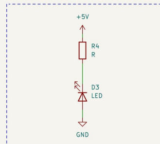
LED témoin de tension
