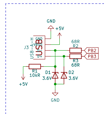
Connecteur USB
